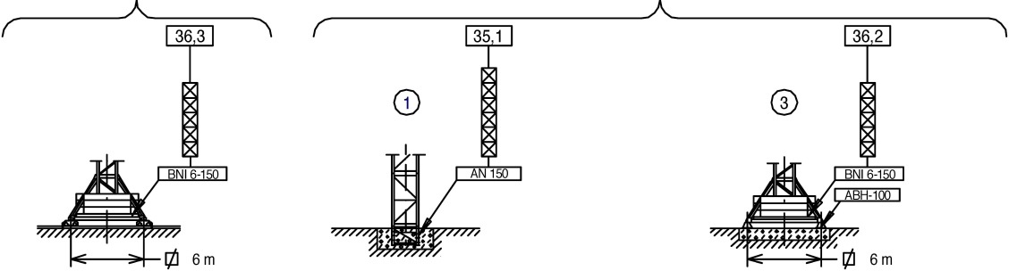
(H) TRASLACION / TRAVELLING / TRANSLATION / ПЕРЕМЕЩЕНИЕ / RAY YÜRÜYÜŞLÜ / متحركة
