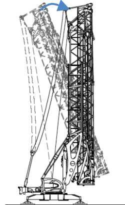
Fin du relevage de la mâture
