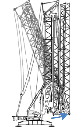
Ouverture et verrouillage de la flèche
