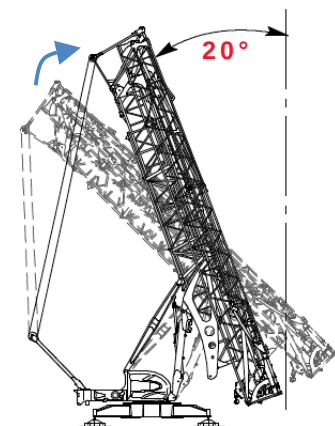
Relevage de la mâture jusqu'à la position 20° (signal sonore)
